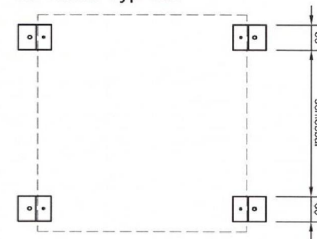
Einbausituation für: Starkstrom-Verteiler Hager Volta AP Breite 305 mm für Kanal Typ 420
